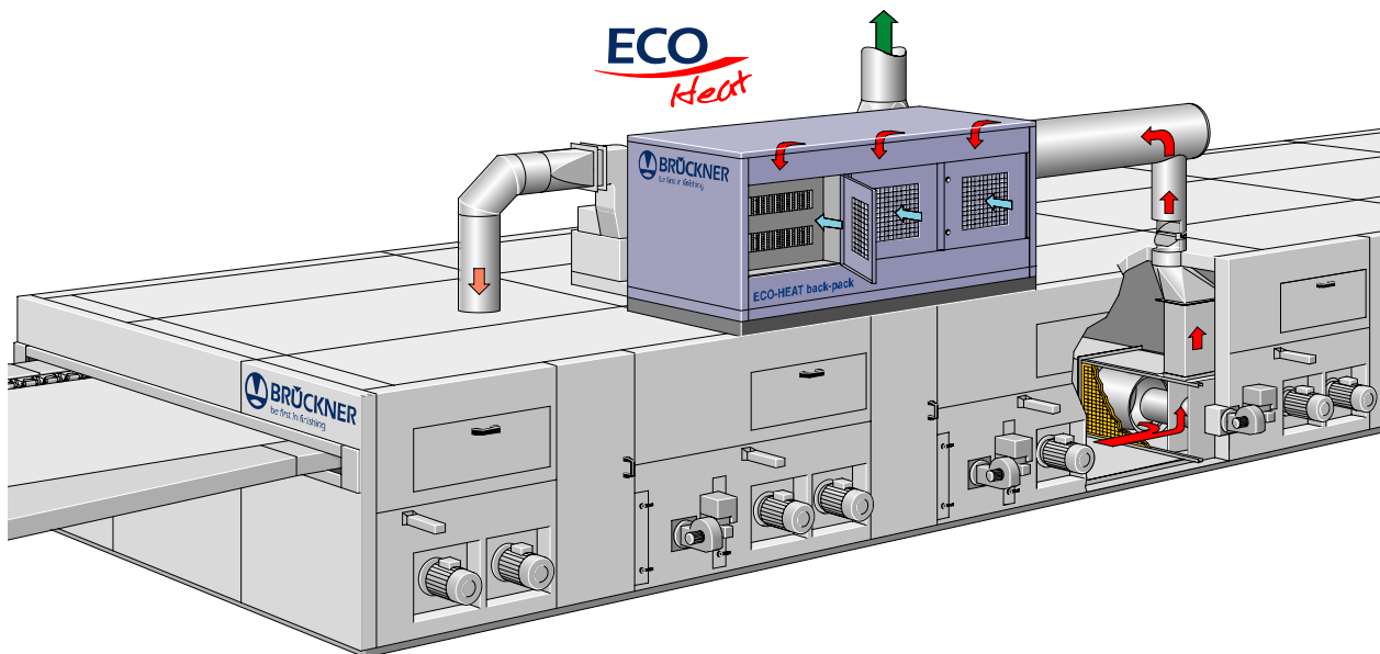
BRÜCKNER Spannmaschine POWER-FRAME mit integrierter Wärmerückgewinnung ECO-HEAT back-pack
